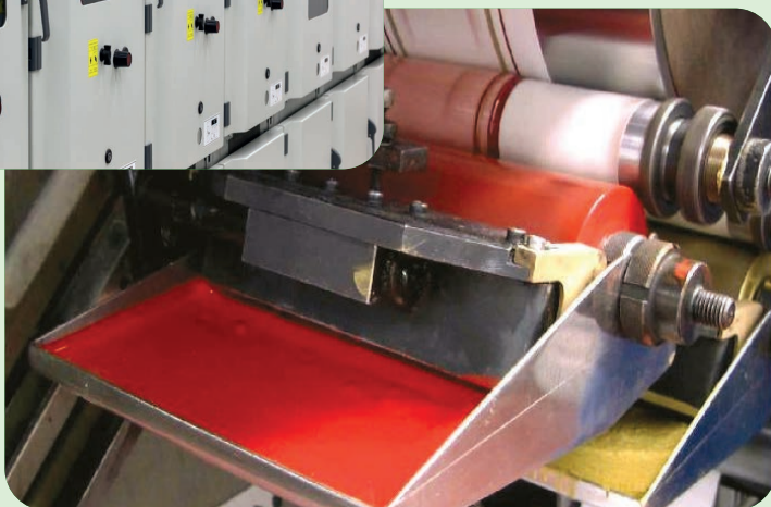
Nettoyage des encres en flexographie.
