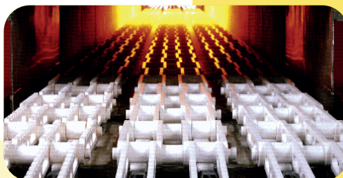
Lubrification d'entraînements de tapis de fours. Cuisson de polymères conducteurs phénoliques/argent à 220 °C en continu.
